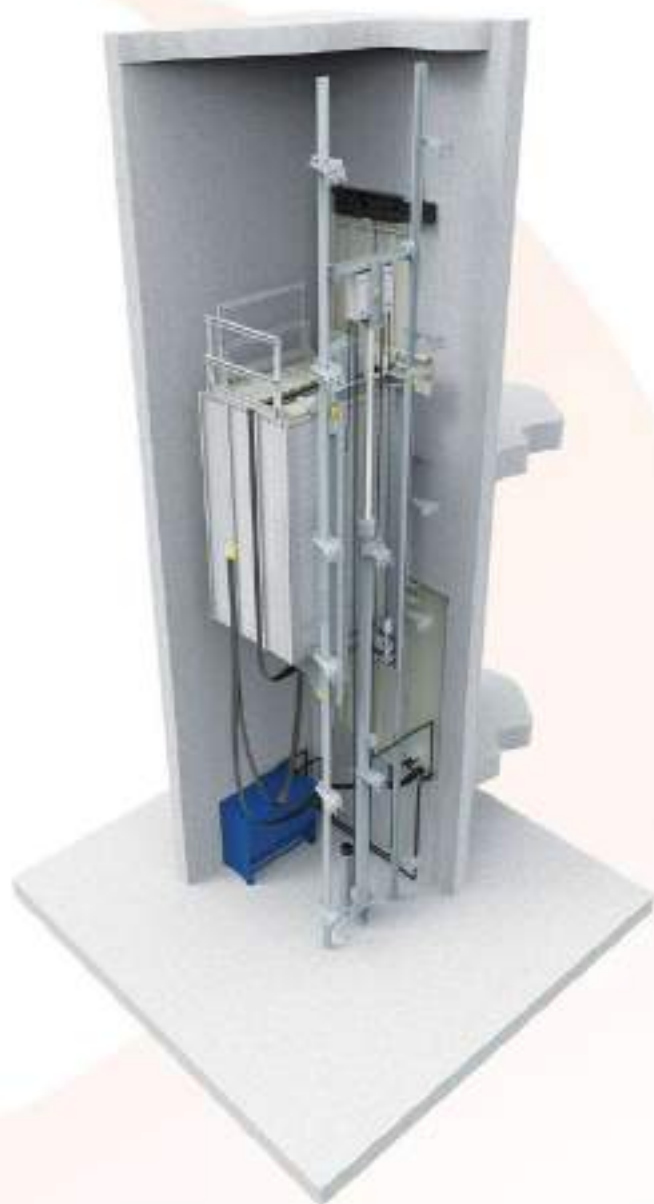
Hidrolik Sistem Hydraulic System Гидравлическая Система نظام المضاعد الهيدروليكية
